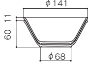
TK-02M ボール 高高台
