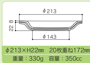
WG-02M リム丸プレート(大)
